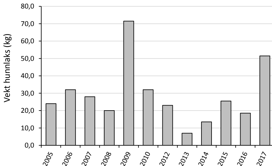
Figur 29. Totalvekt av hunnlaks (gytebiomasse) beregnet fra data fra gytefisktelling i innløpselva til Urvodvatnet i årene 2005 til 2017. I 2011 ble det ikke gjennomført drivtelling.
