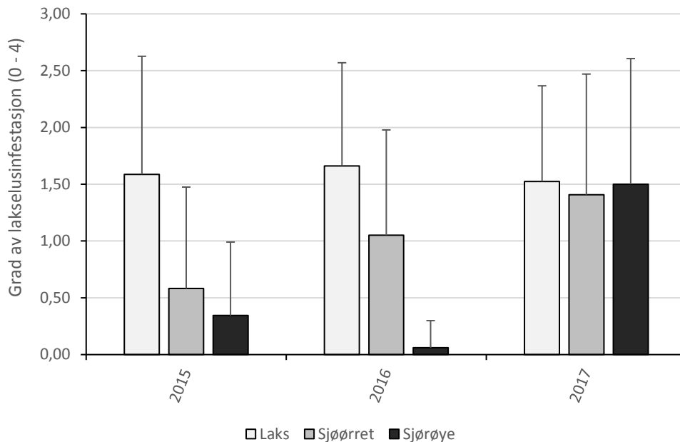
Figur 27. Graden av lakselusinfestasjon registrert på laks, sjørørret og sjørøye beregnet fra resultater fra videoovervåkningen på Ureidet i Urvoldvassdraget i årene 2015 til 2017.
