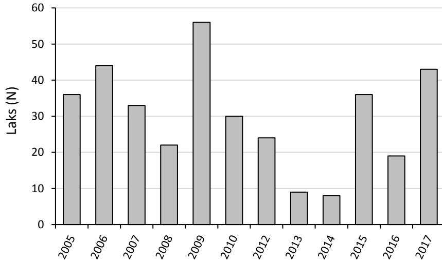
Figur 28. Antall laks registrert under gytefisktelling i innløpselva til Urvodvatnet i årene 2005 til 2017. I 2011 ble det ikke gjennomført drivtelling.
