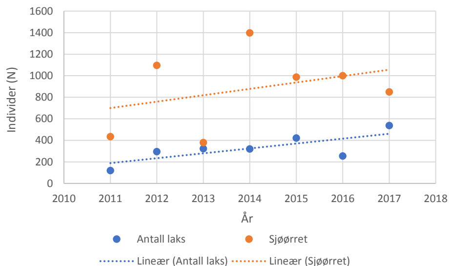
Figur 8. Antall sjørørret og laks registrert under drifttelling i Åelva i årene 2011 til 2017 i forhold til år. Det er kun tatt med år der hele elvestrekningen er undersøkt.
